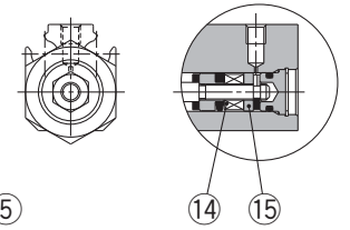
Eingebauter Magnetring
